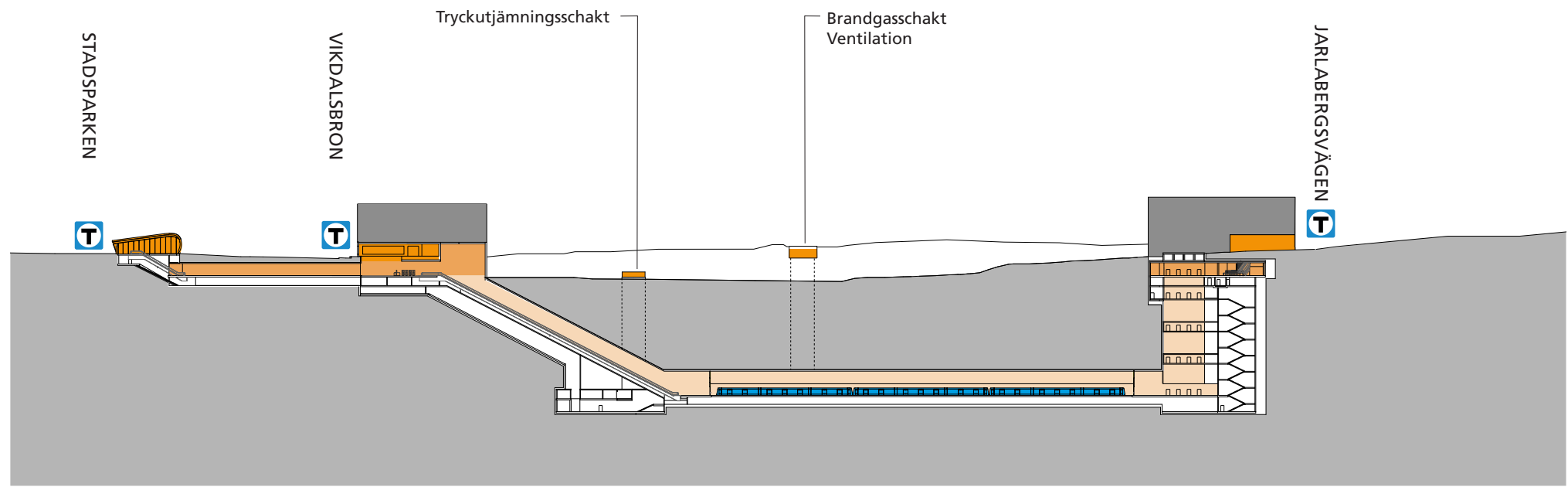
Längdsektion
