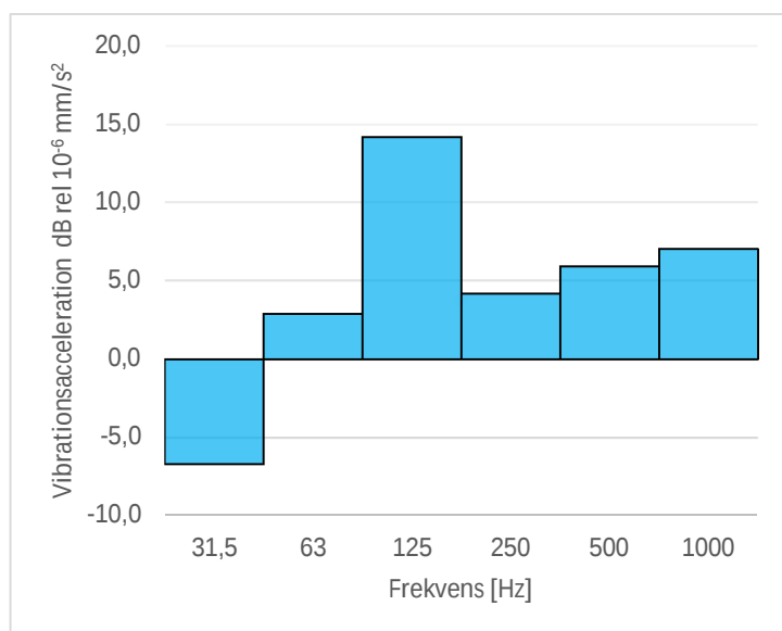
Figur 9 Dämpning i ett elastiskt mellanlägg under spår jämfört med ballasterat spår utan stomljusdämpande åtgärder
