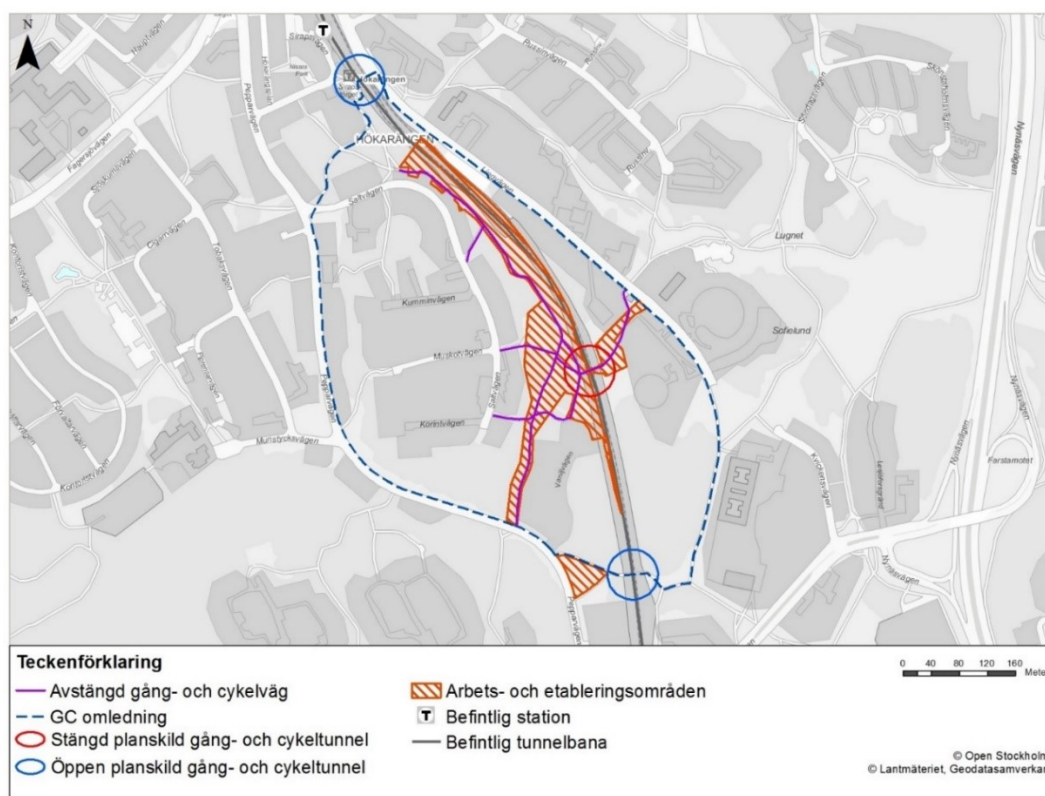
Figur 31. Befintliga gång- och cykeltunnlar vid anslutning till Farstagrenen som är öppna och stängda under byggskedet.
