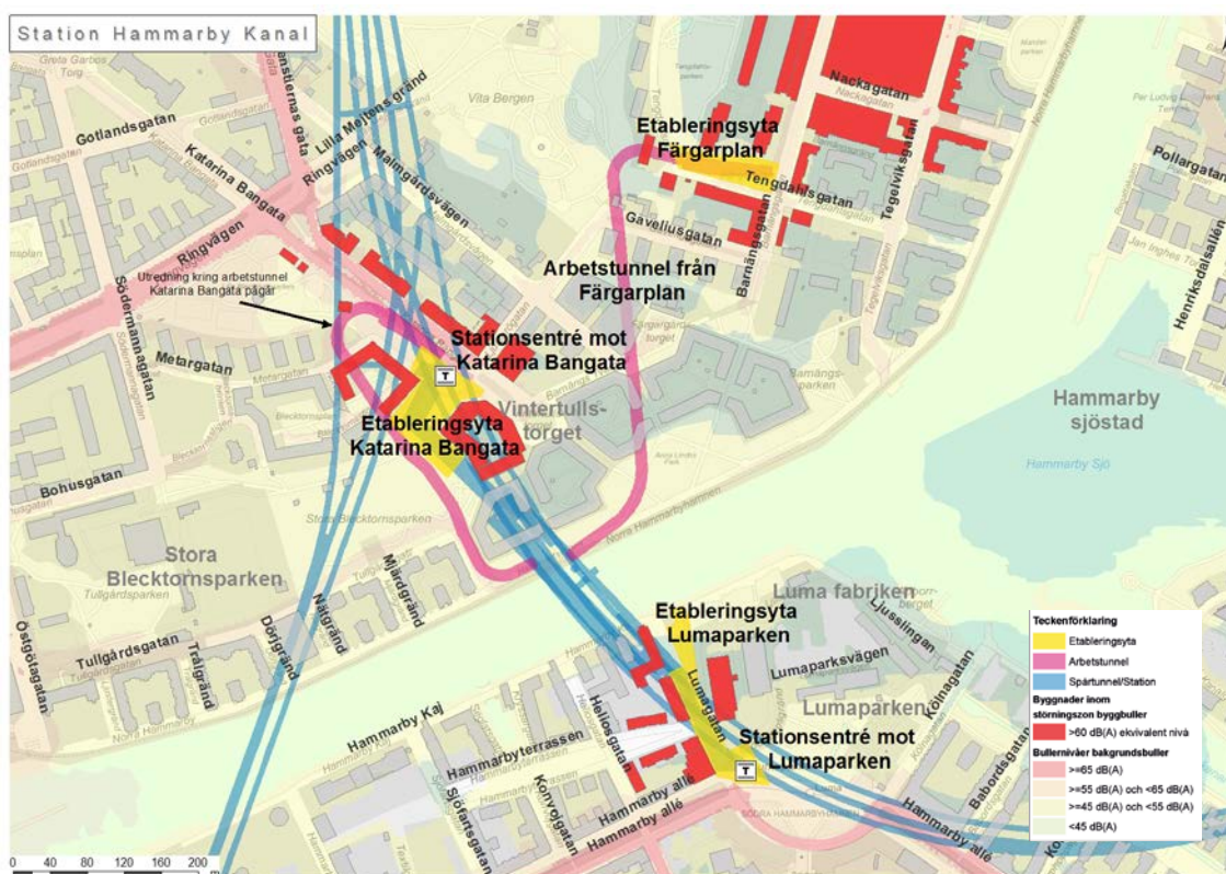
Figur 31. Bullerspridning av byggbuller vid station Hammarby Kanal
