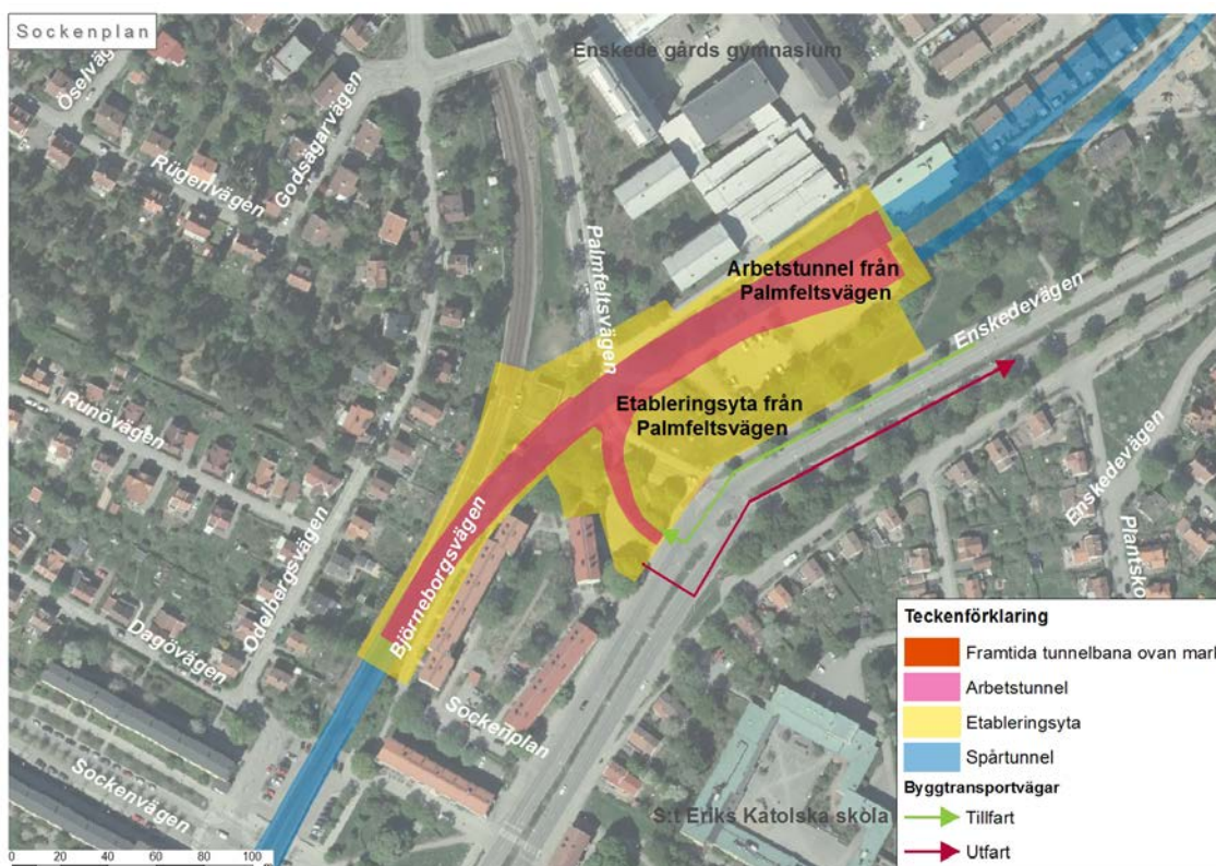
Figur 52. Karta över anslutning Sockenplan
