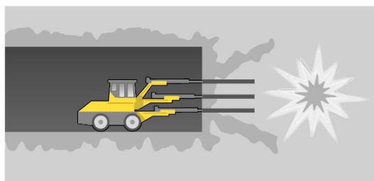
1-5 meter långa hål borras för sprängning och laddas sedan med sprängmedel. Sprängningen sker i etapper enligt ett bestämt mönster för att minimera vibrationerna.
