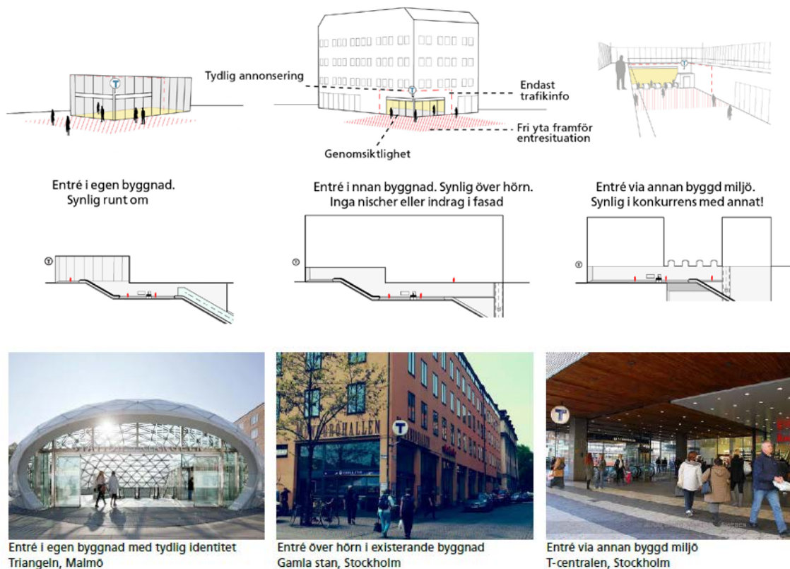
Figur 8. Skiss över station med entré i egen byggnad, i annan byggnad eller via annan byggd miljö och foton från motsvarande i Malmö och Stockholm.
