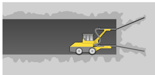
Injektering: Cementbruk pumpas in i borrhål och bergssprickor. När den stelnat bildas en tätning runt den blivande tunneln.
