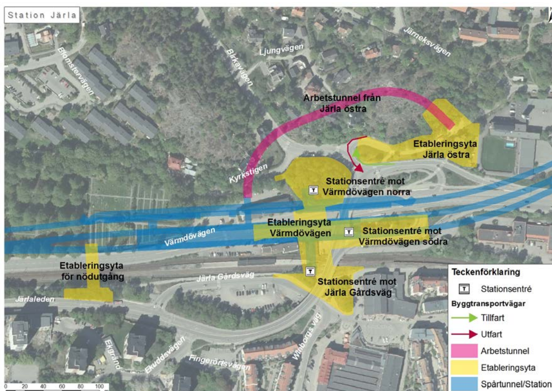
Figur 37. Karta över station Järla. Etableringsyta Järlaleden krävs för byggande av nödutgång.
